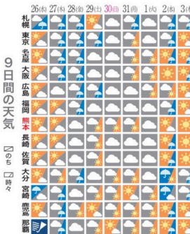
9日間の天気
